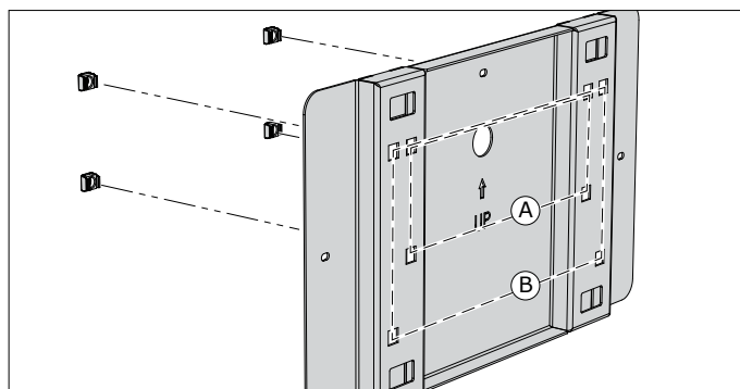
Fig. 4.1 Cage nuts
