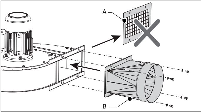
Fig. 4.19 Fan outlet transition
