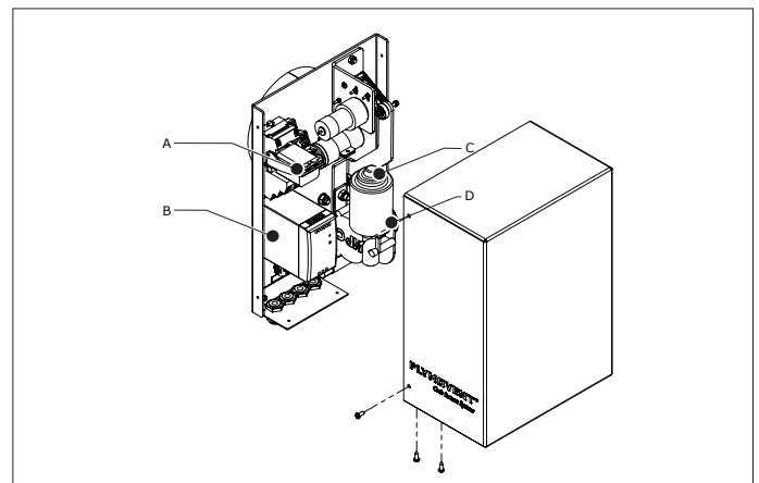
Fig. 10.1 Spare parts
