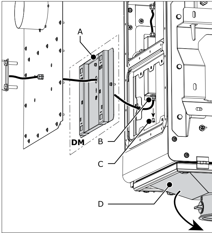
Fig. 4.11 Raccordement du câble
