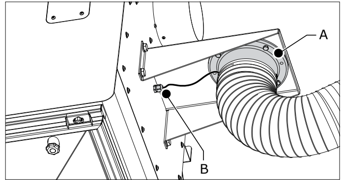
Fig. 4.10 Passe-fil + presse-étoupe de câble
