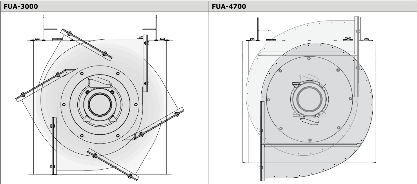
Fig. III Directions possibles de la sortie du ventilateur
