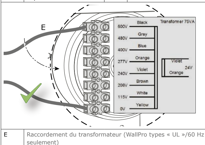
Fig. 4.16 Coffret électrique
