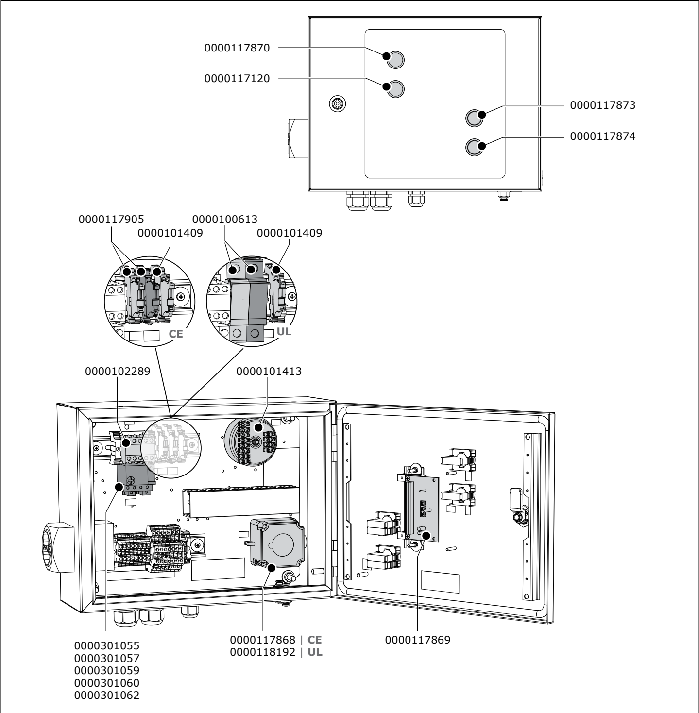
Fig. X Vue éclatée du coffrret électrique
