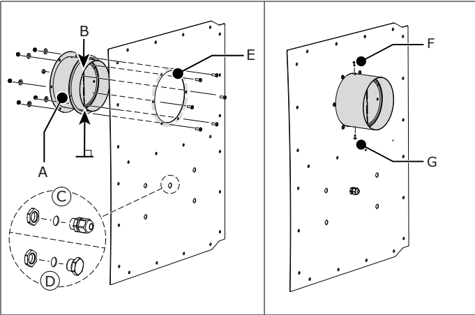
Fig. 4.3 Bride d'entrée + clapet anti-retour (ensemble)
