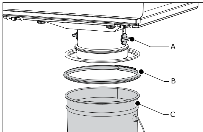
Fig. 6.4 Vidage du bac à poussière
