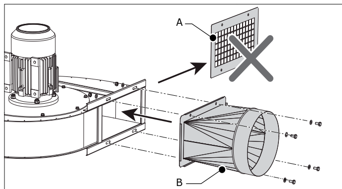
Fig. 4.19 Pièce de raccordement du ventilateur
