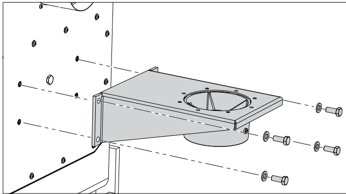
Fig. 4.5 Montage du support de bras
