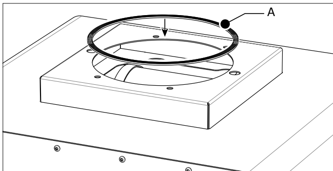
Fig. 4.6 Bande caoutchouc adhésive
