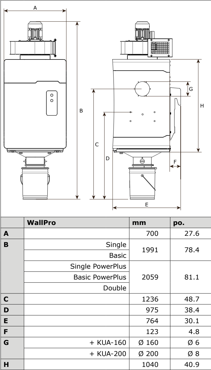
Fig. I Dimensions
