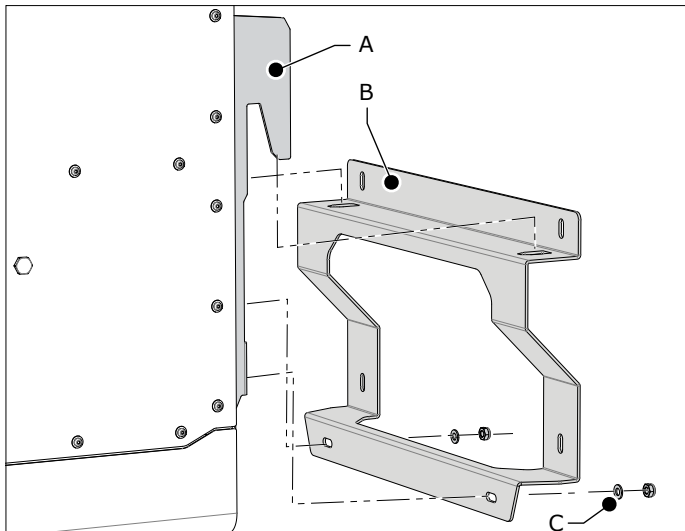
Fig. 4.9 Montage du support mural
