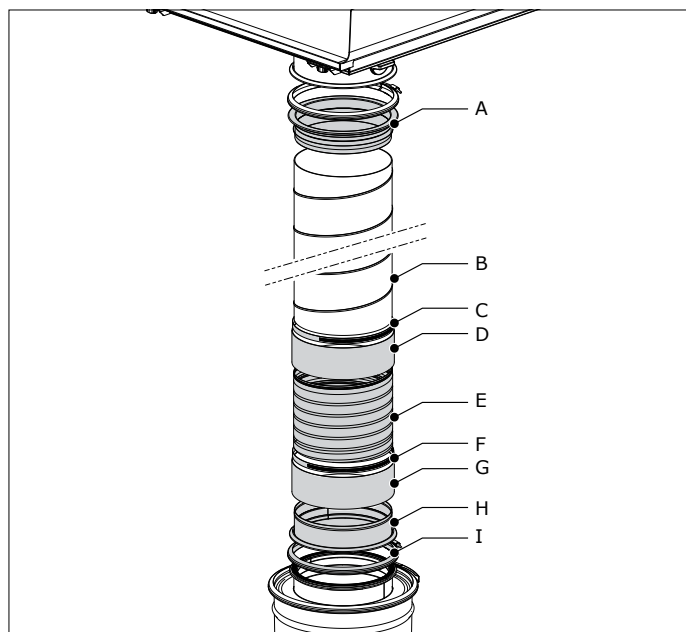
Fig. 4.15 Jeu d'extension pour le bac à poussière
