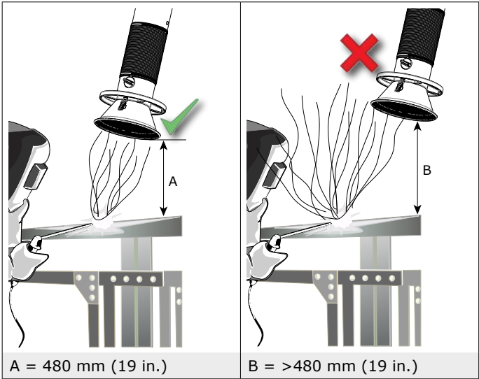
Fig. VII Positionnement du bras d'aspiration
