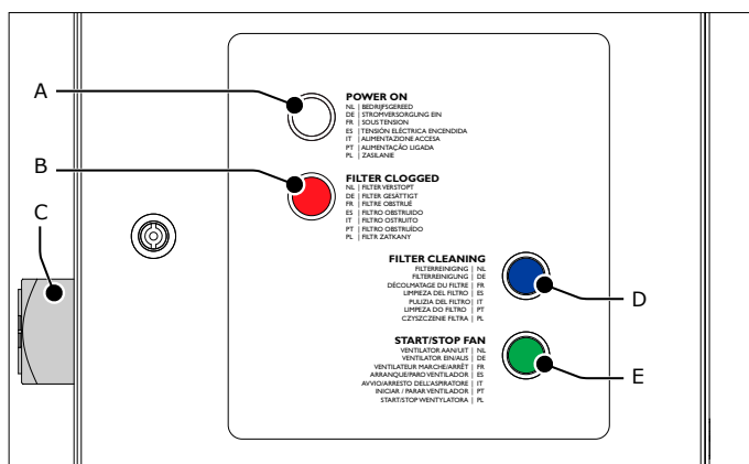
Fig. 5.1 Tableau de commande
