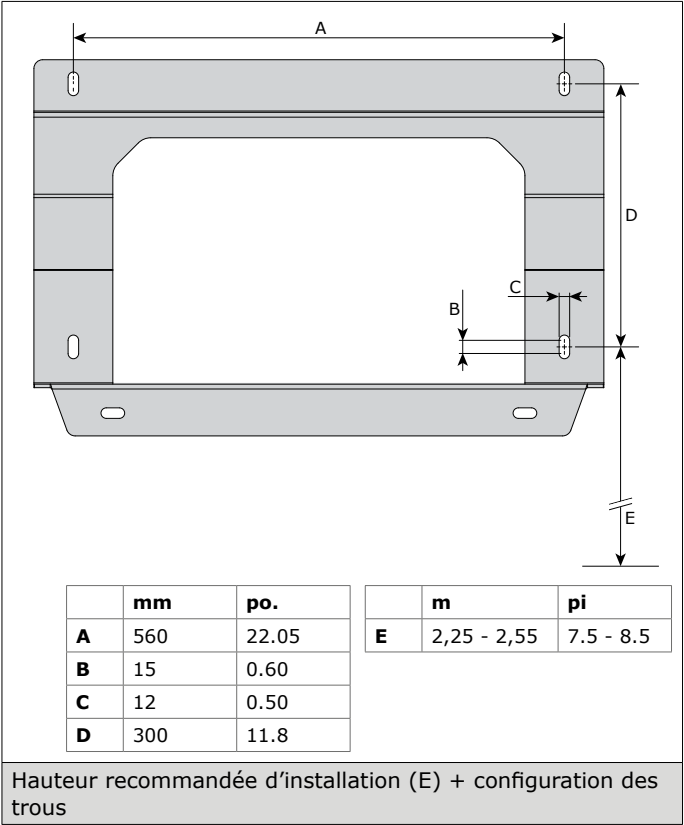
Fig. VI Hauteur d'installation
