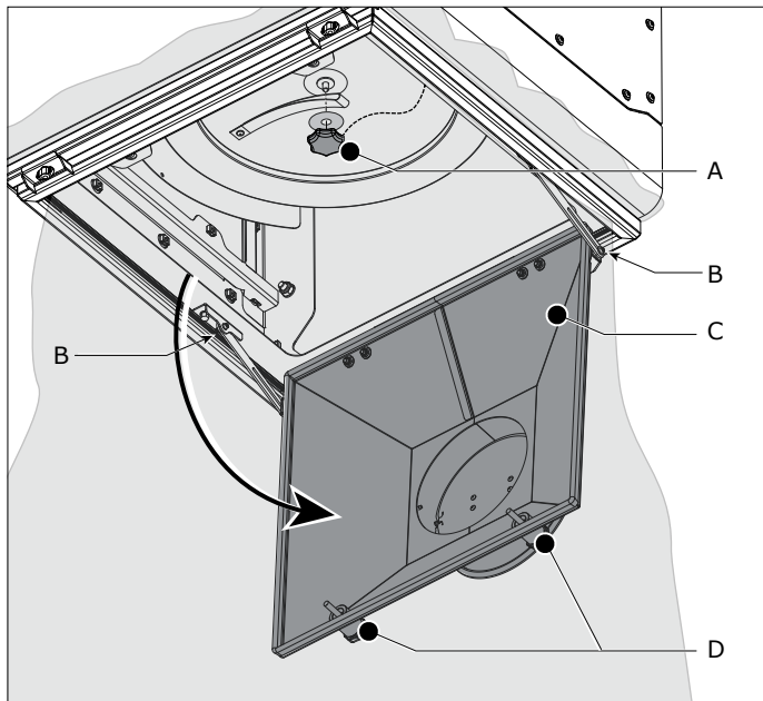
Fig. 6.3 Remplacement de la cartouche filtrante
