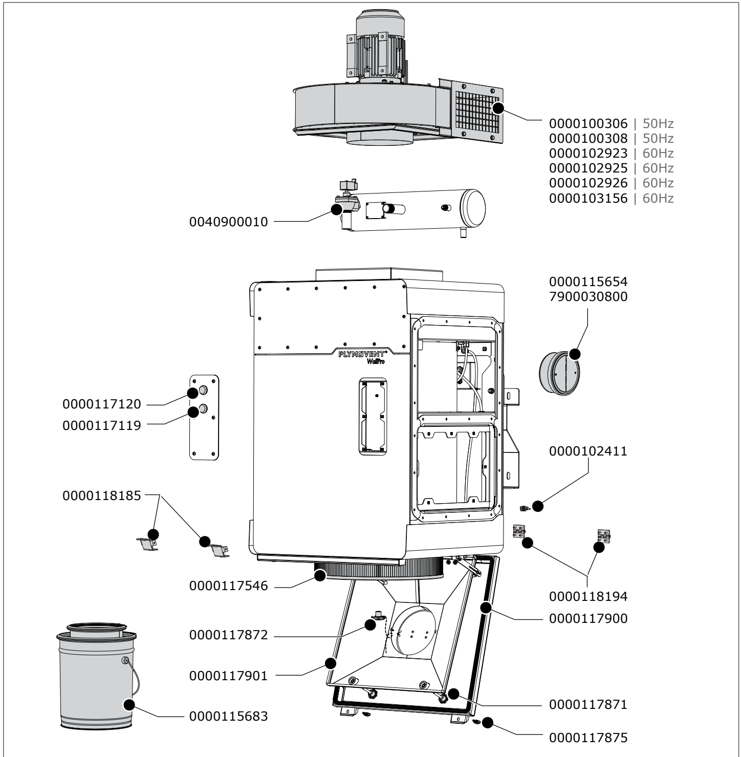
Fig. IX Vue éclatée de l'unité de filtration (WallPro)
