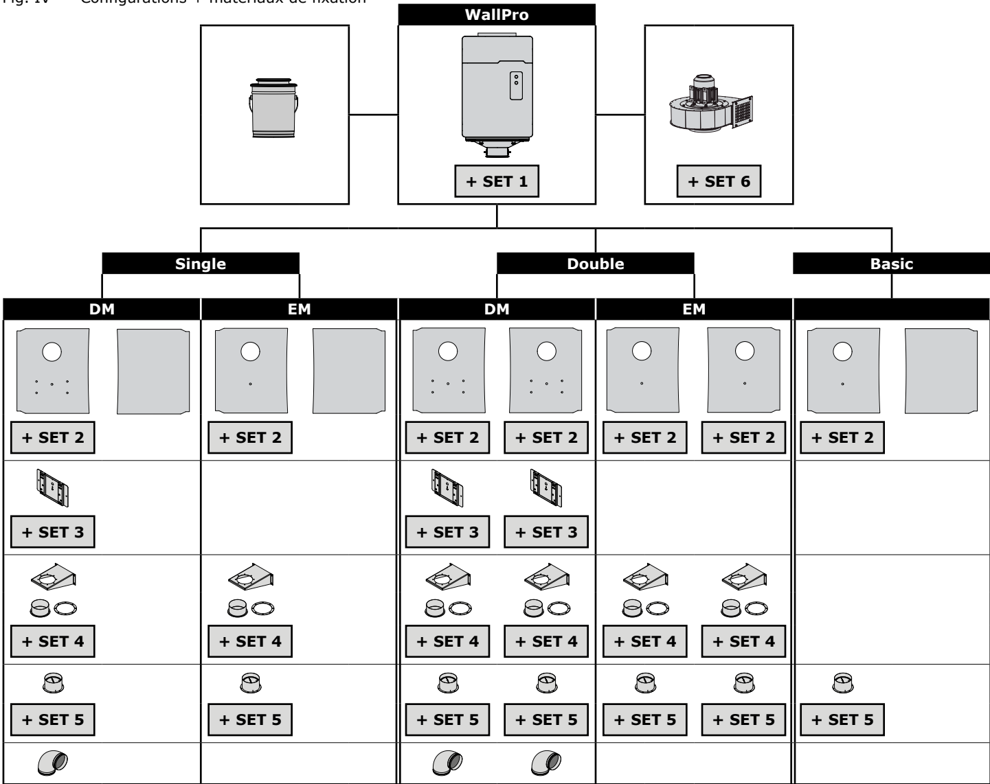
Fig. IV Configurations + matériaux de fixation
