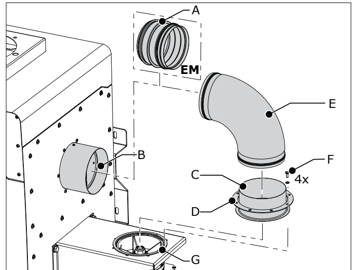
Fig. 4.13 Conduite d'entrée
