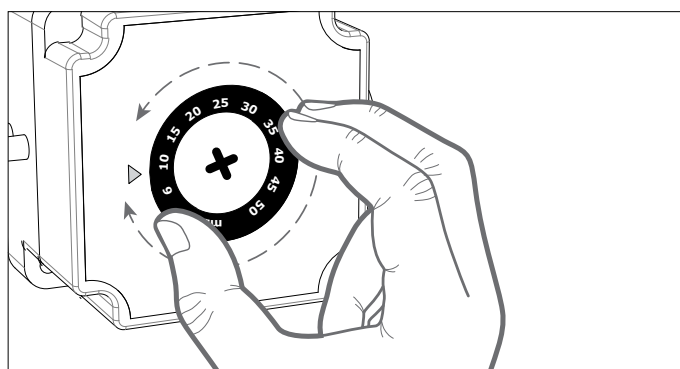
Fig. 4.18 Commutateur différentiel
