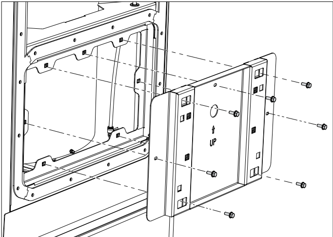
Fig. 4.2 Montage de la plaque de renfort
