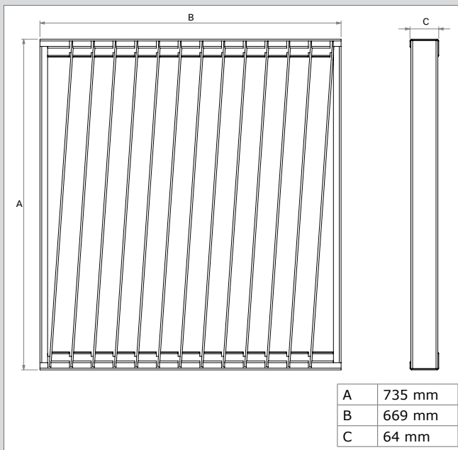
Arbetsgaller för plasmaskärning galler (topp och sidovy)
