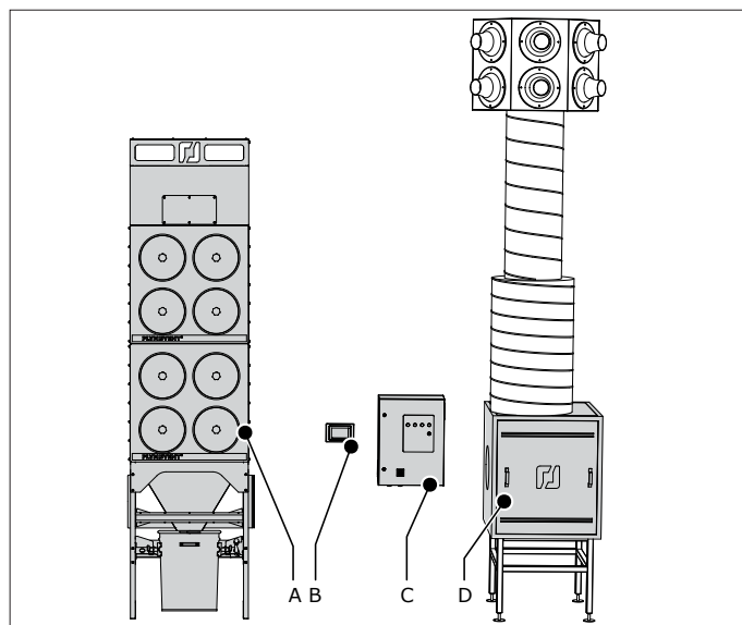
Fig. 1.1 MDB-Diluter PRO
