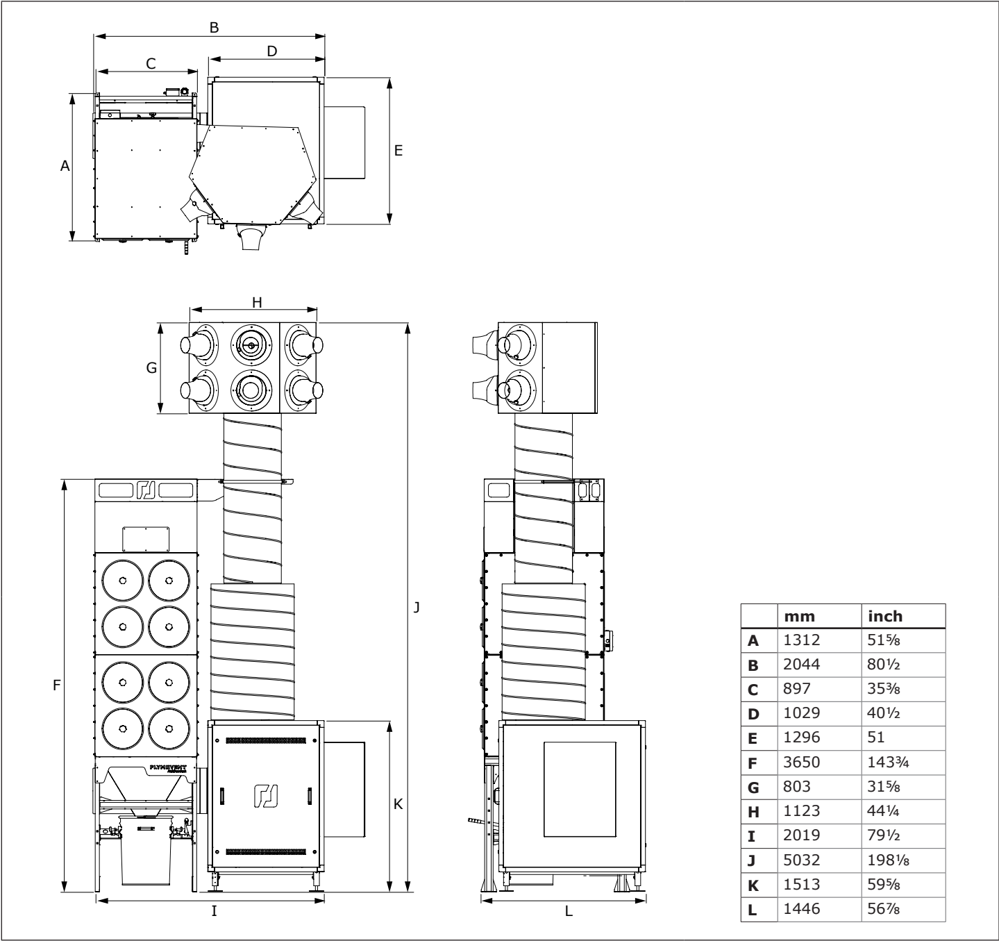
Fig. I Dimensions MDB-Diluter
