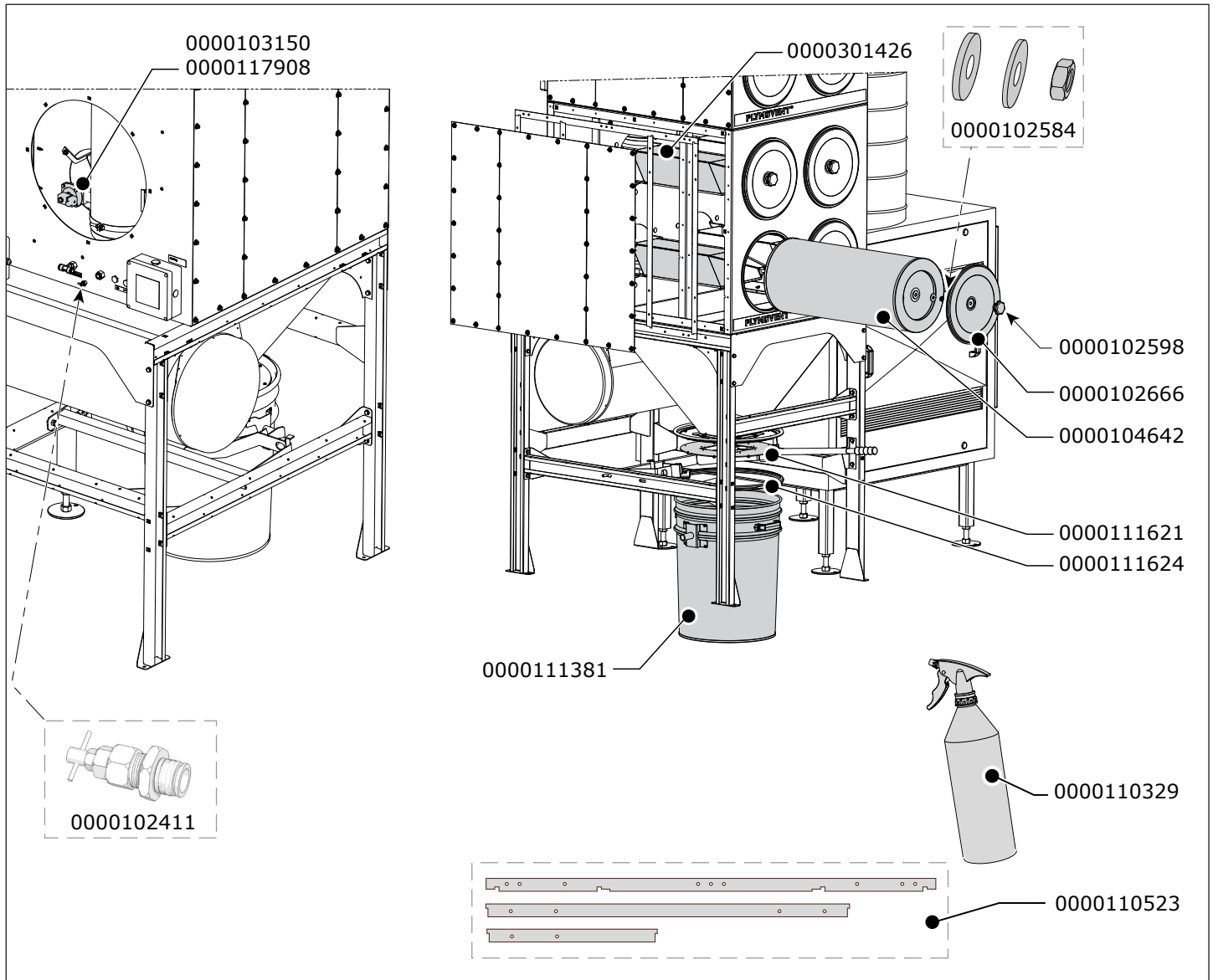
Fig. VII MDB-Diluter
